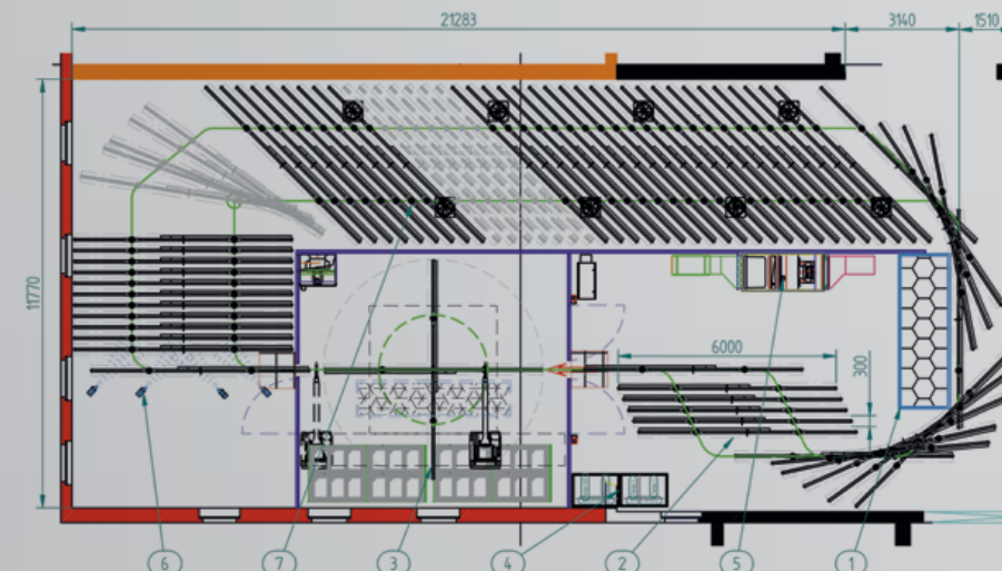
Beispiel 02: Lackieranlage mit Roboter für die Holzfensterbeschichtung
