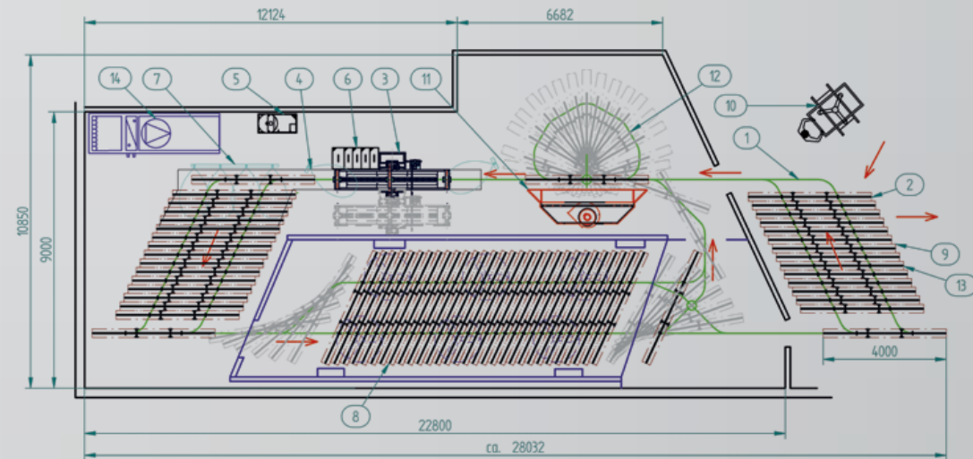
Beispiel 01: Flut- und Lackieranlage für Holzfenster
